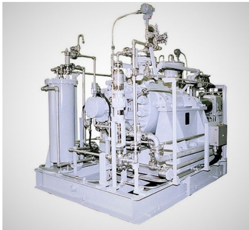
《参考画像》今回納入予定機器と同型式のポンプ及び駆動用蒸気タービン
